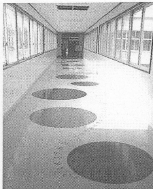
円・円周率
