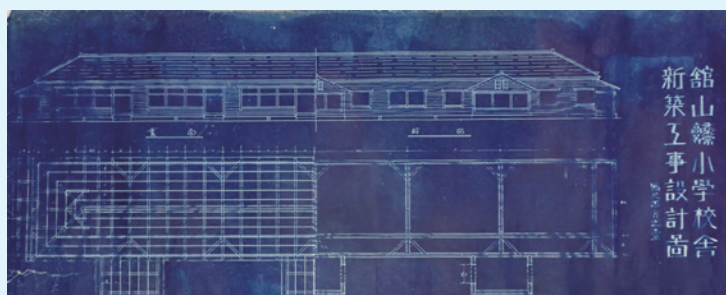
館山小学校舎設計図
