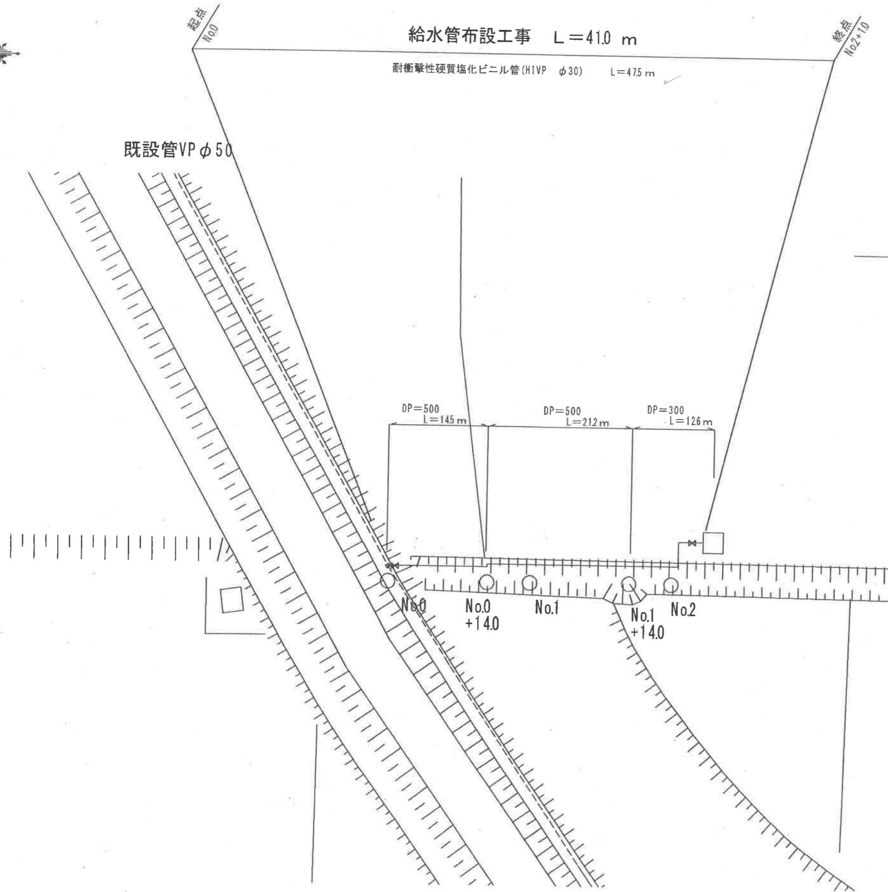
平面図 S 1:500
