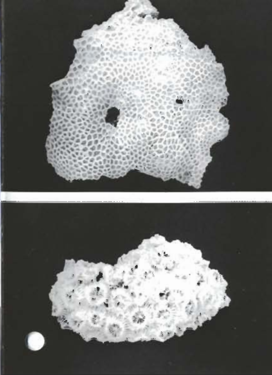
沼サンゴ層産の造礁性サンゴ化石
