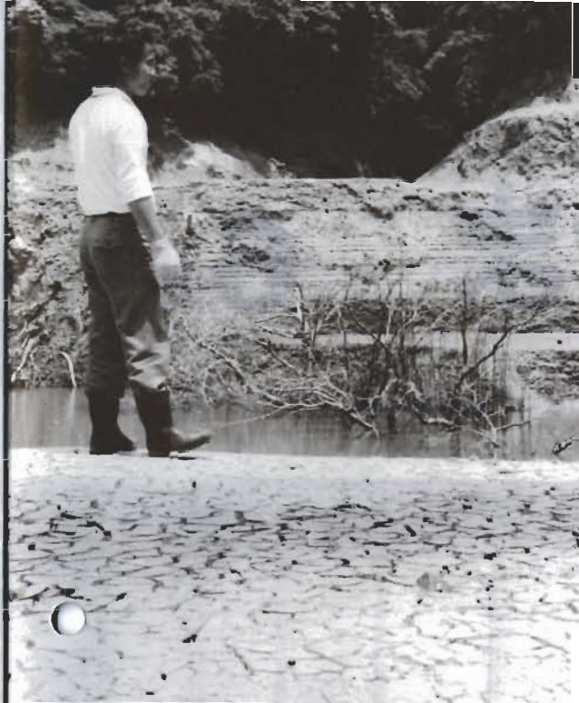
ダム底にヒビ割れが…(増間ダム)
