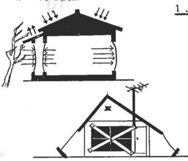
家に対する風圧
