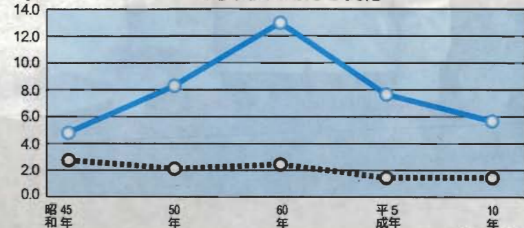
▼汐入川のBOD変化
