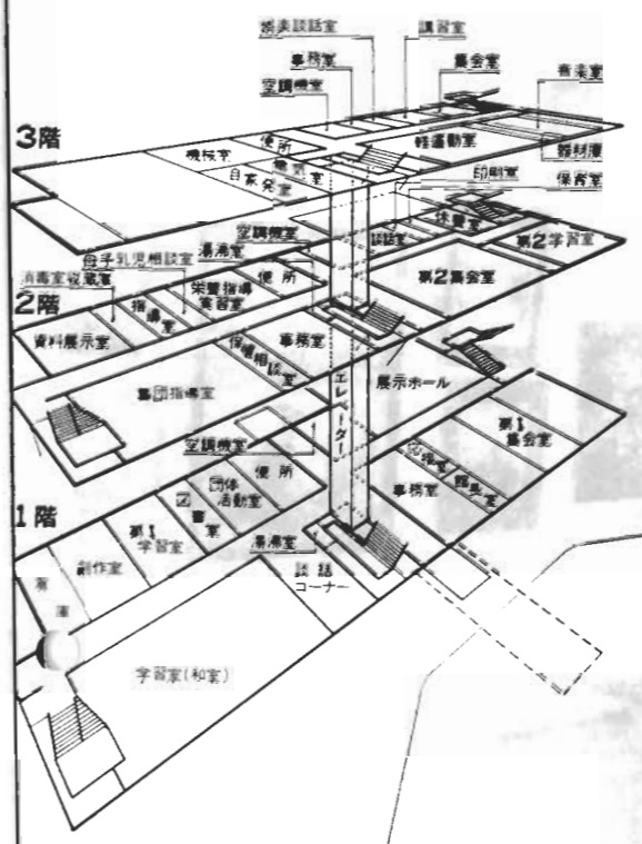
館山市コミュニティセンター案内図
